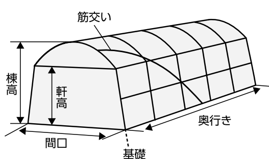
図１ ハウスの構造
