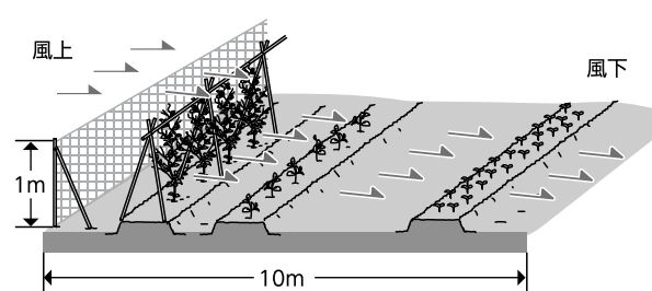
図2 防風ネットの設置
